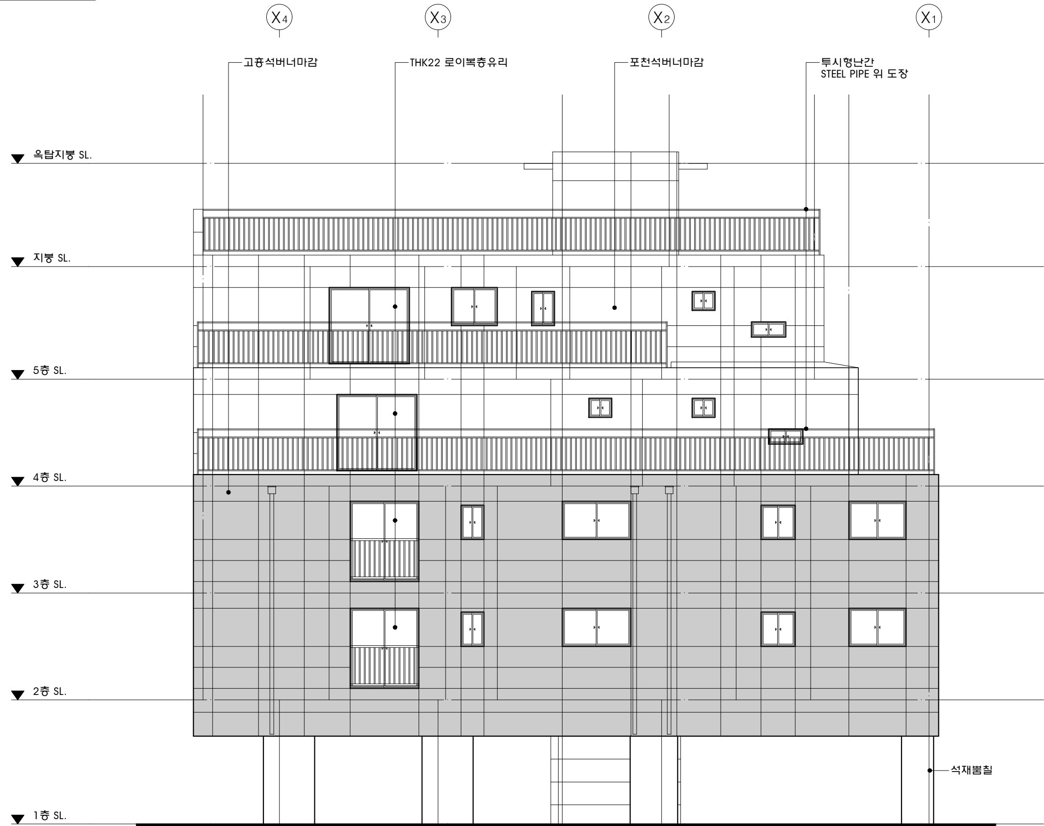
1 우측면도 축척 - A3 : 1/100
